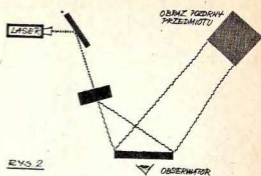
Rys. 2. Odtwarzanie hologramu
